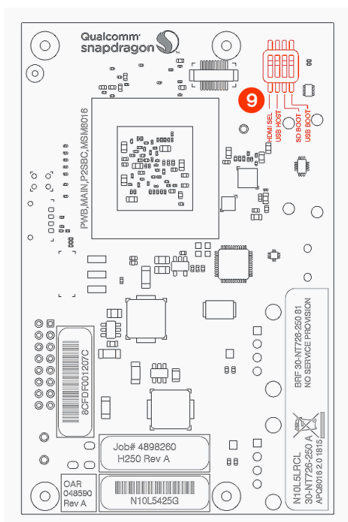
図 4. ボード裏面
