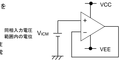
Figure 56. 未使用回路の処理例
