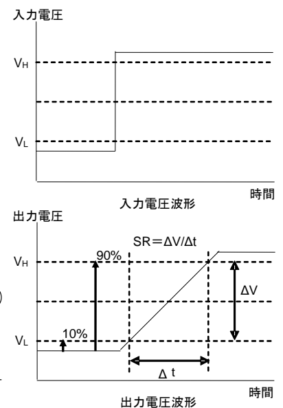
Figure 50. スルーレート測定時波形
